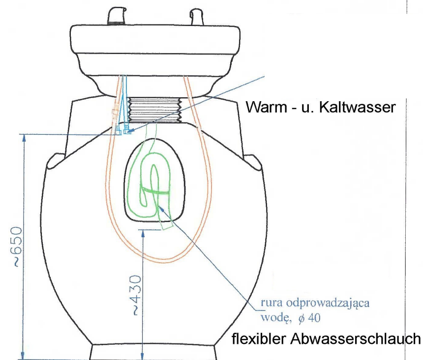
Anschlusszeichnung
